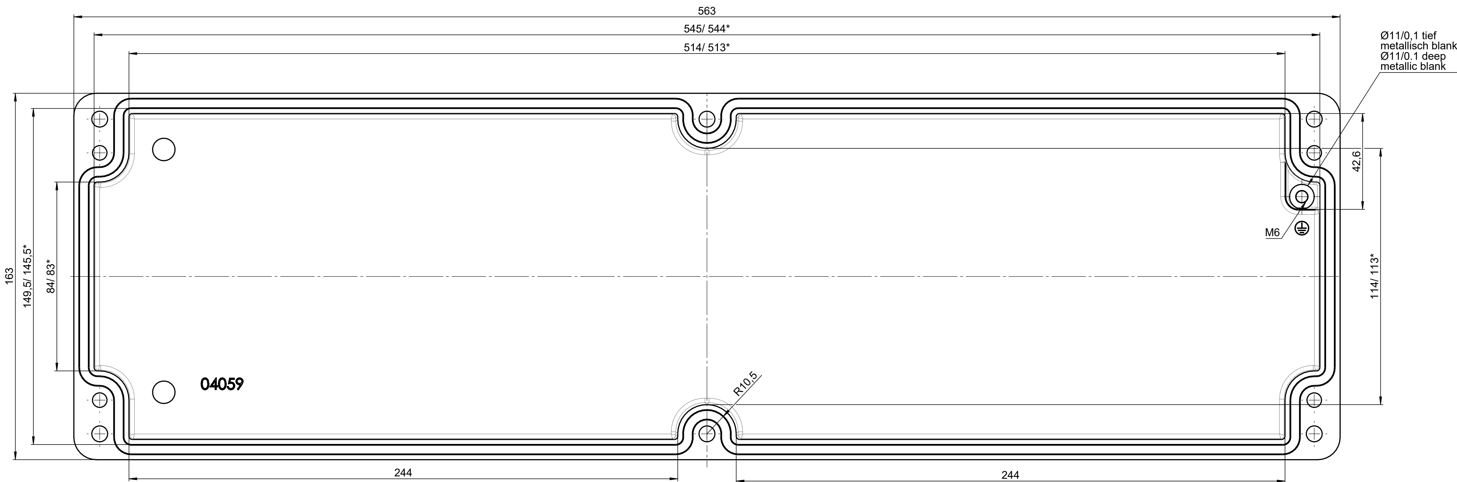
Deckel / Lid
